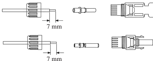
Obr. 3.3 Demontáž krytu matice konektoru
