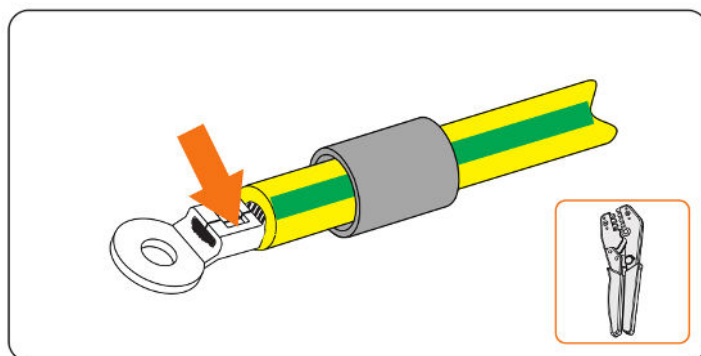
Zakrmpování kabelového oka
